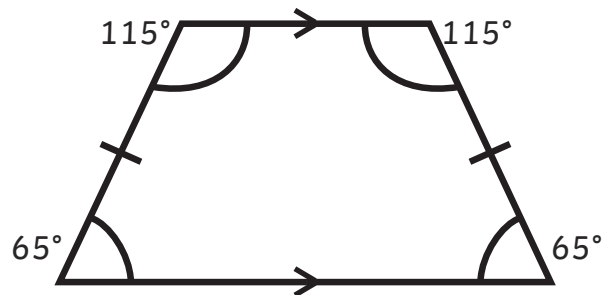
Isosceles Trapezium
