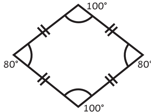
Rhombus
